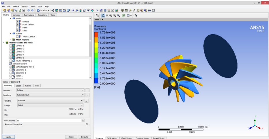
Figura 11. Presión sobre la microturbina.
