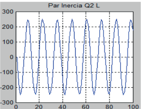
Figura 11. Par Inercia Q2 obtenido por Lagrange.
