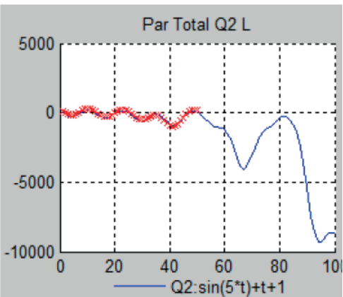
Figura 9. Par Total Q2 obtenido por Lagrange.
